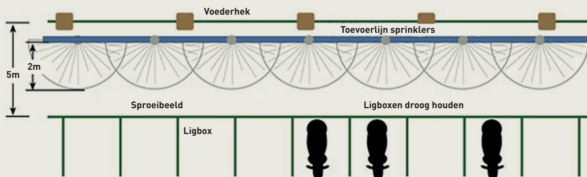
Figuur 3. Plaatsing en sproeibeeld sproeiers aan voederhek
